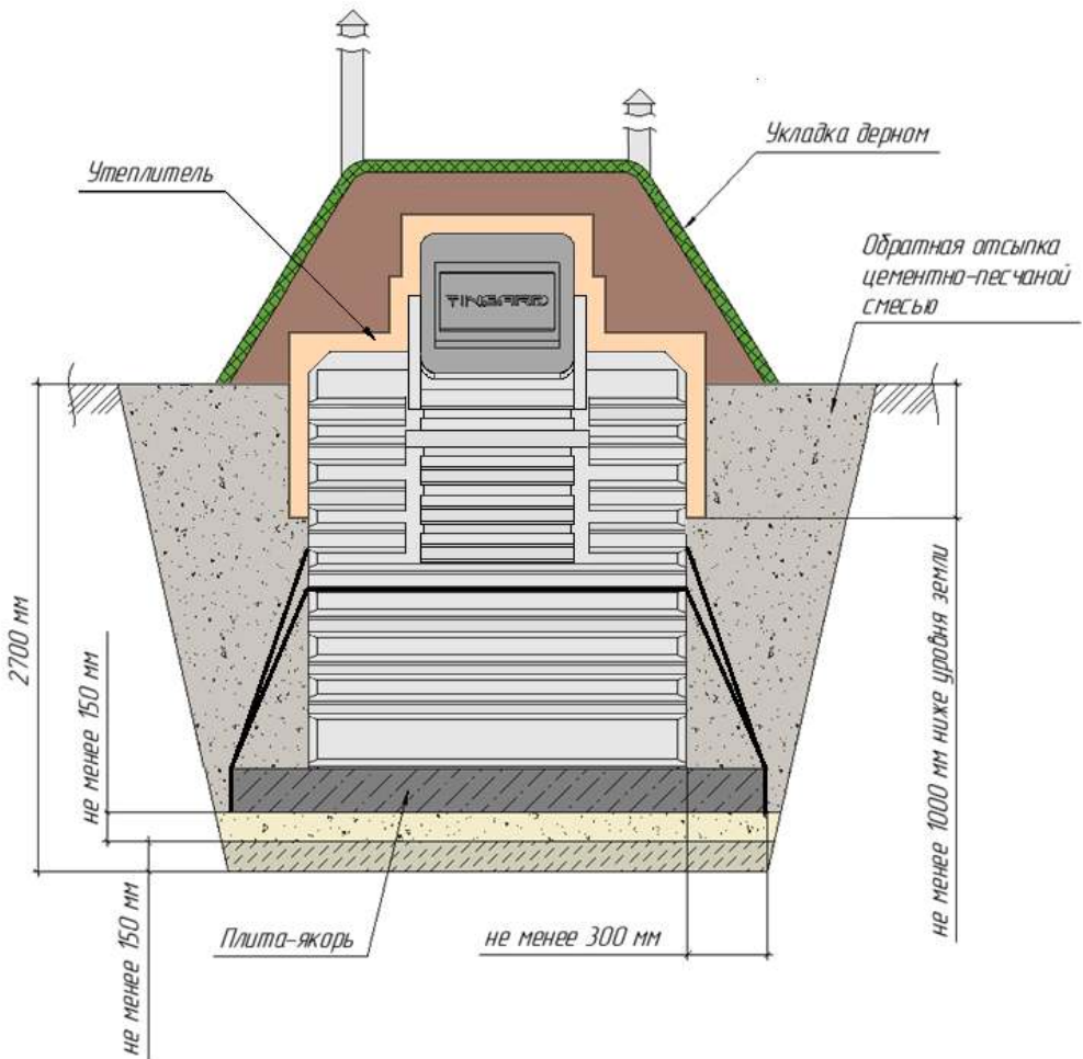
Схема монтажа погреба Т1900БК, Т2500БК
