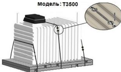
Рисунок 6. Схемы якорения погребов
