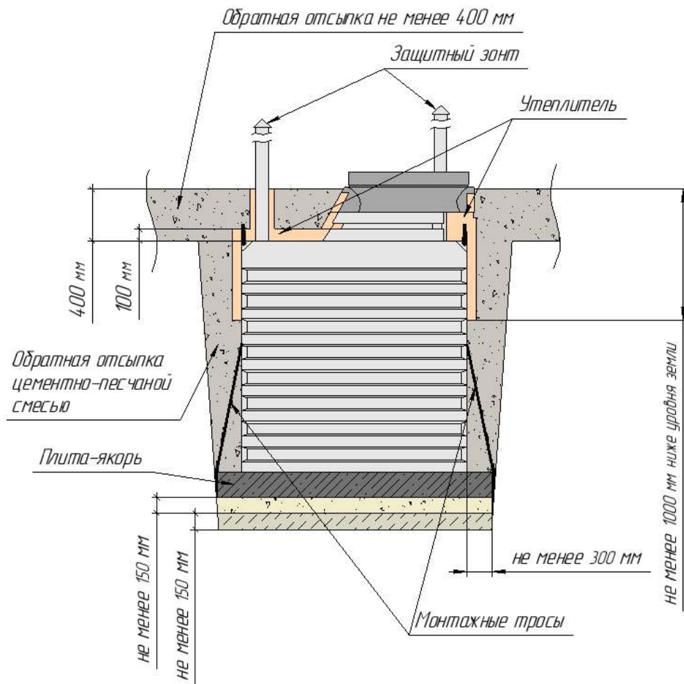
Схема монтажа погреба Т3000-3500 с нижним якорением
