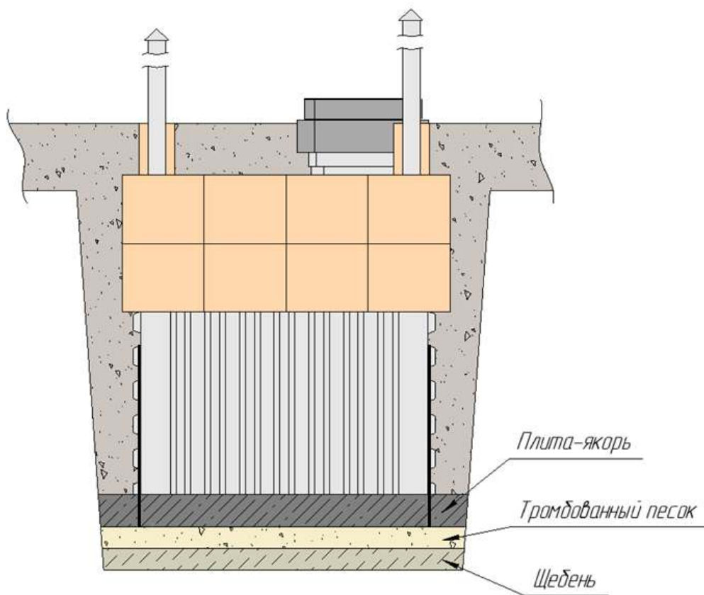
Схема монтажа погреба Т1900-2500 с нижним якорением
