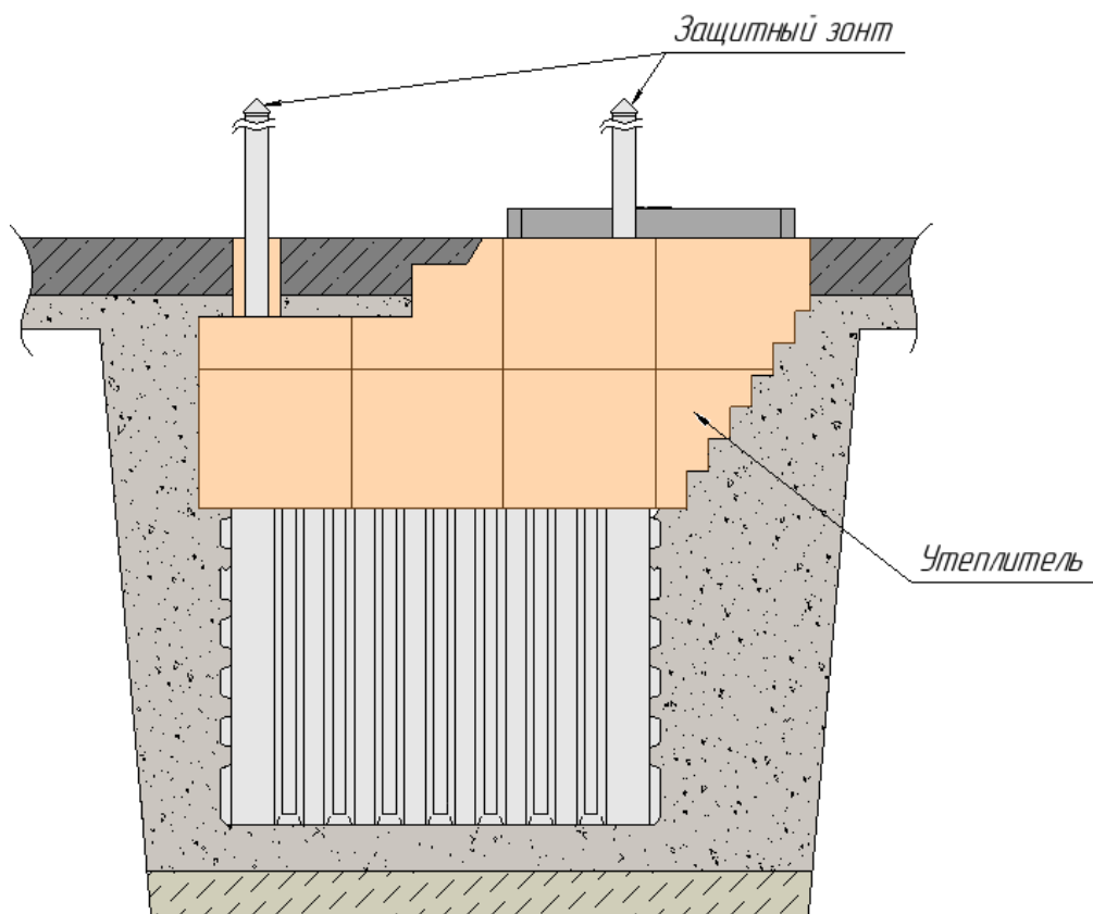
Схема монтажа погреба Т1900К, Т2500К с верхним якорением
