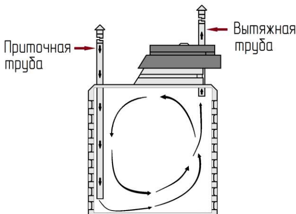
Рисунок 7. Схема циркуляции воздуха в приточно-вытяжной вентиляции.
