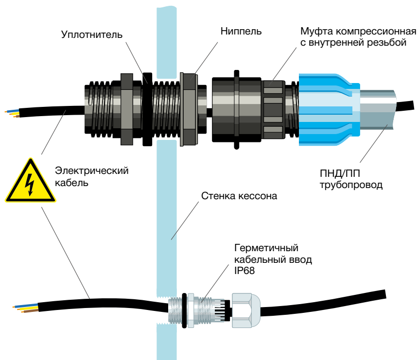
Варианты монтажа эл. кабеля внутрь кессона Еврослос
